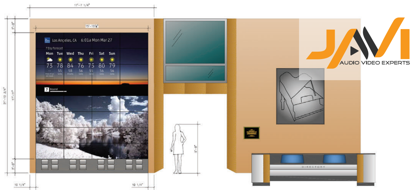
1 VIDEO WALL ELEVATION – (4x8 SAMSUNG UH55F-E) SCALE: N.T.S.
